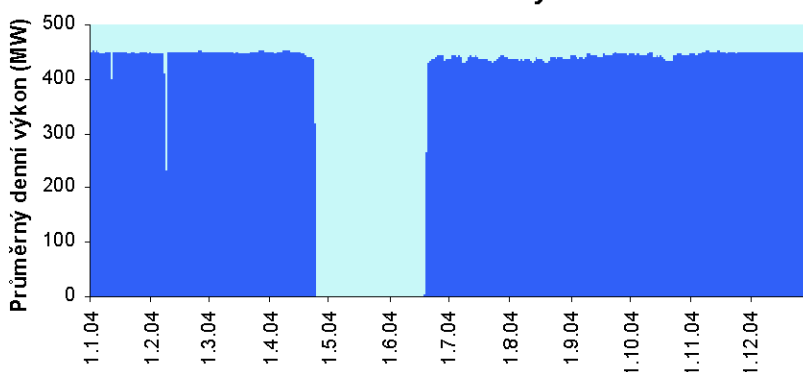
2. blok JE Dukovany
