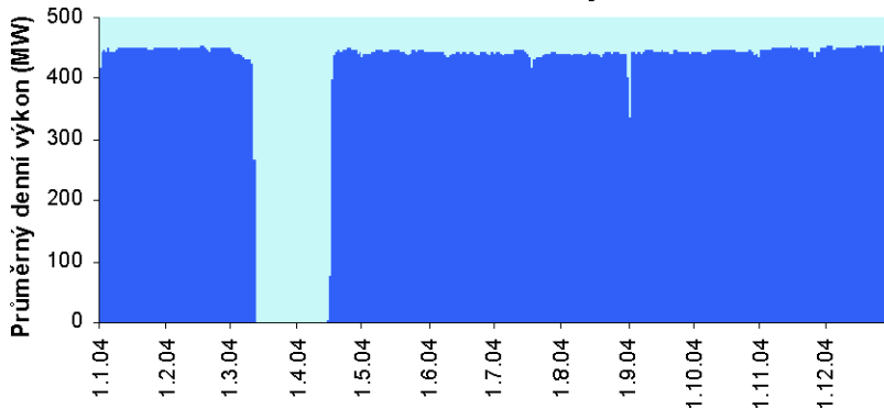
3. blok JE Dukovany
