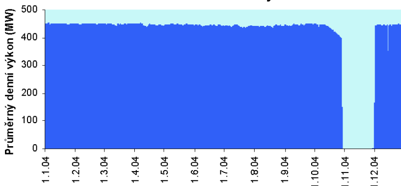
4. blok JE Dukovany
