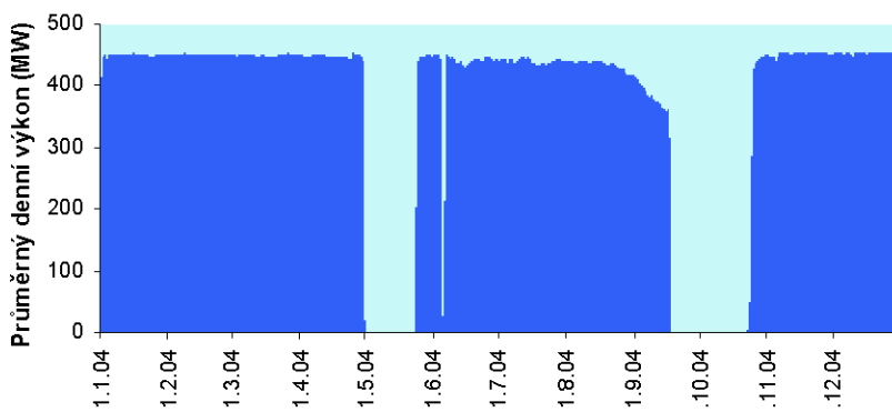
1. blok JE Dukovany
