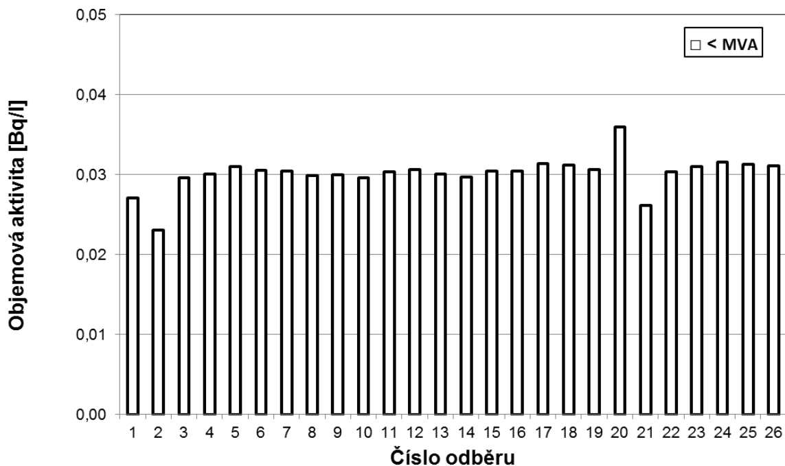
Obr. 18a Objemová aktivita ^{137}\text{Cs} v mléce v roce 2016 ve vzorcích odebraných v kravínech v ZHP JE Dukovany (odebírání se jednou za 14 dní; odběr a měření LRKO JE Dukovany)
