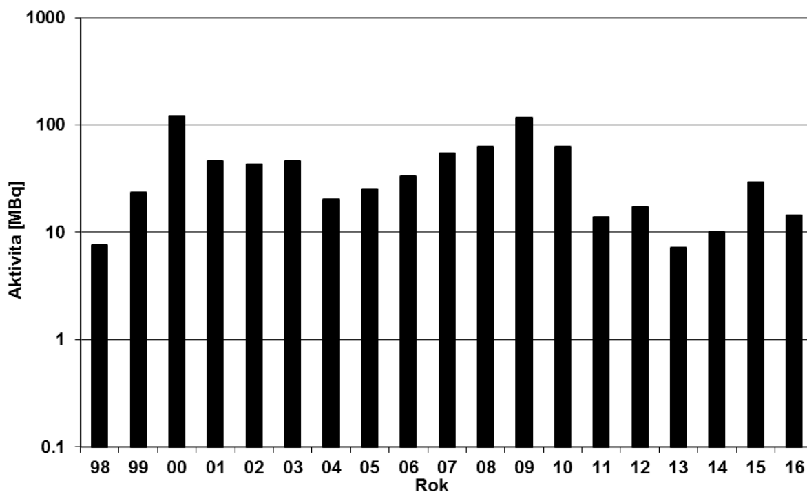
Obr. 15b Bilance plyných výpustí - ^{131}\text{I} z odběrů ve ventilačním komínu ÚJV Řež v období 1998 – 2016 (celkový roční limit aktivity je 20 000 [MBq]), (vzorkování a měření ÚJV Řež)
