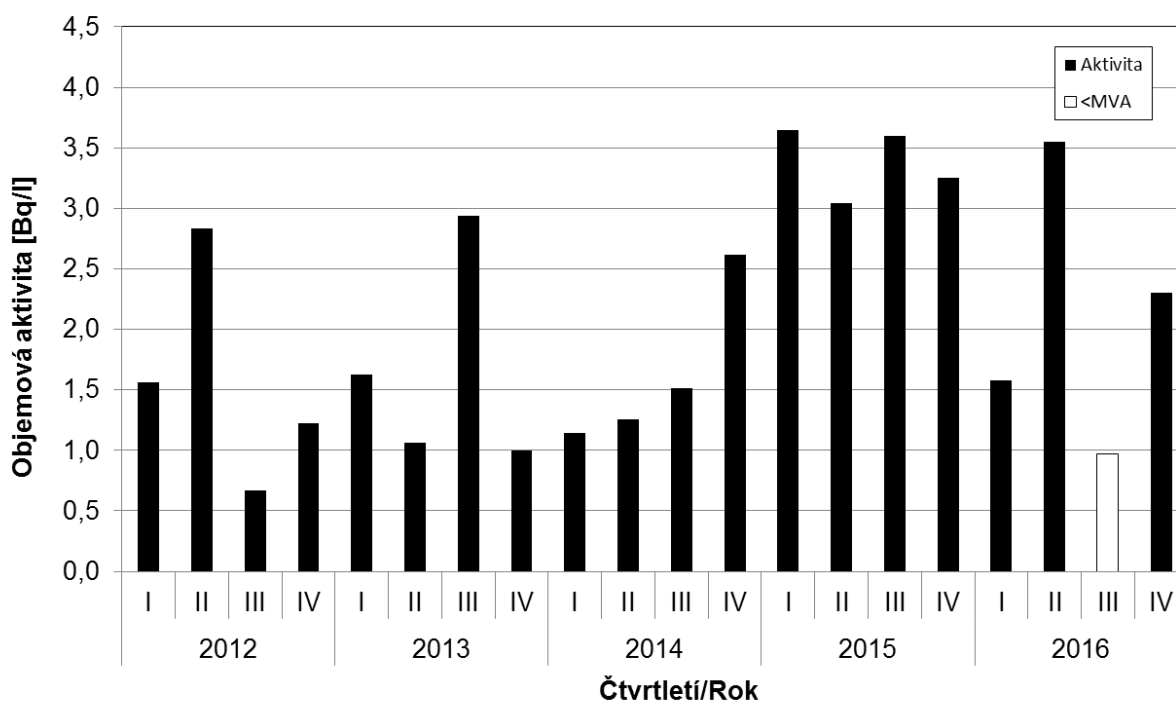
Obr. 12b Objemová aktivita ^3\text{H} v povrchové vodě za posledních 5let – povodí Morava – profil Lanžhot (Morava) (odběrové místo je Moravský Svatý Ján; vzorkování Povodí, s.p., měření VÚV TGM Praha)
