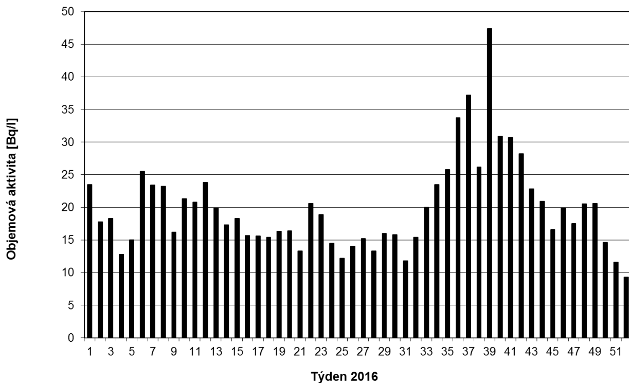
Obr. 12c Objemová aktivita ^3\text{H} v povrchové vodě v roce 2016 – povodí Vltava – profil Praha-Podolí (Vltava) (vzorkování Povodí, s.p., měření VÚV TGM Praha)
