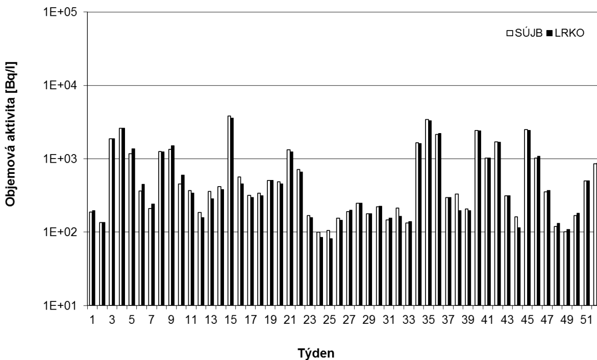
Obr. 19b Objemová aktivita ^3\text{H} v odpadním kanále JE Dukovany v roce 2016 (porovnání hodnot naměřených SÚJB a LRKO provozovatele, odběr JE Dukovany, měření RC SÚJB Brno a LRKO JE Dukovany)
