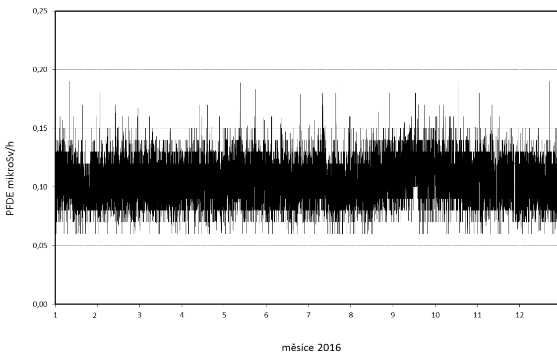
Obr. 16a Příkon fotonového dávkového ekvivalentu (PFDE) - SVZ TDS1 Dukovany (měřicí místo č. 18)
