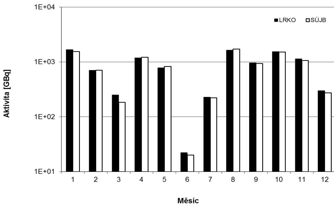
Obr. 19a Celková aktivita ^3\text{H} vypouštěná do vodoteče z JE Dukovany v roce 2016 (porovnání hodnot naměřených SÚJB a LRKO provozovatele, odběr JE Dukovany, měření RC SÚJB Brno a LRKO JE Dukovany)
