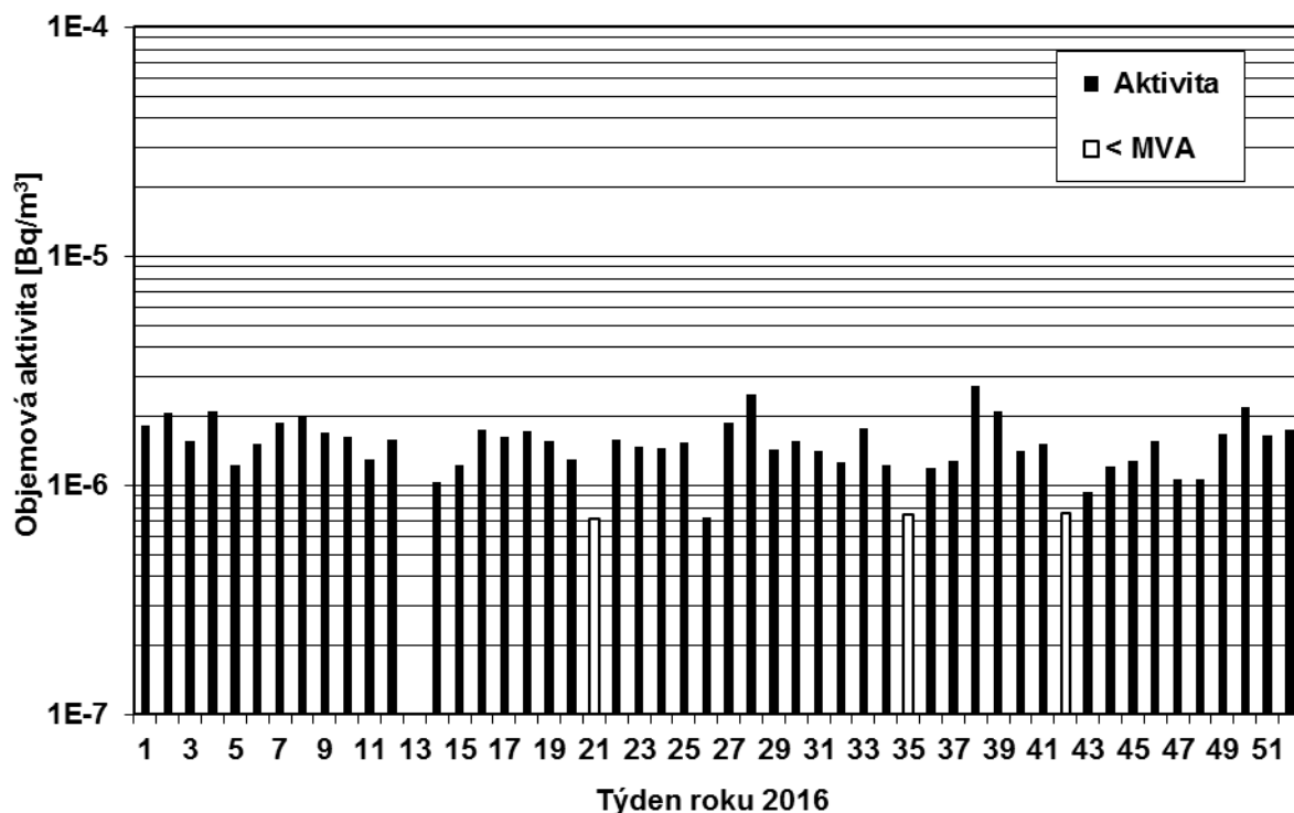
Obr. 7b Objemová aktivita 137 Cs v aerosolu v ovzduší v roce 2016 – MMKO Plzeň (vzorkování MMKO Plzeň, měření RC SÚJB České Budějovice)
