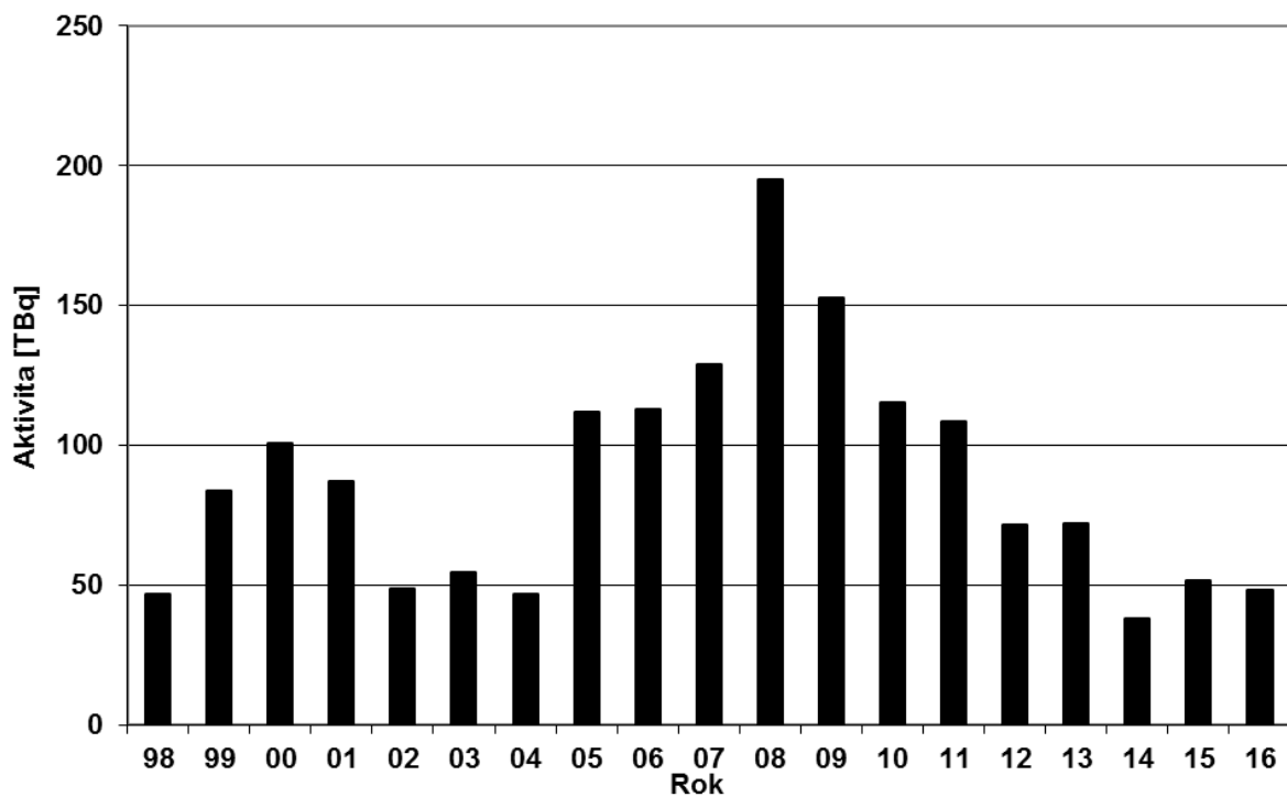
Obr. 15a Bilance plyných výpustí – vzácné plyny ( 41 Ar) z odběrů ve ventilačním komínu ÚJV Řež v období 1998 – 2016 (celkový roční limit aktivity je 1 000 [TBq]), (vzorkování a měření ÚJV Řež)
