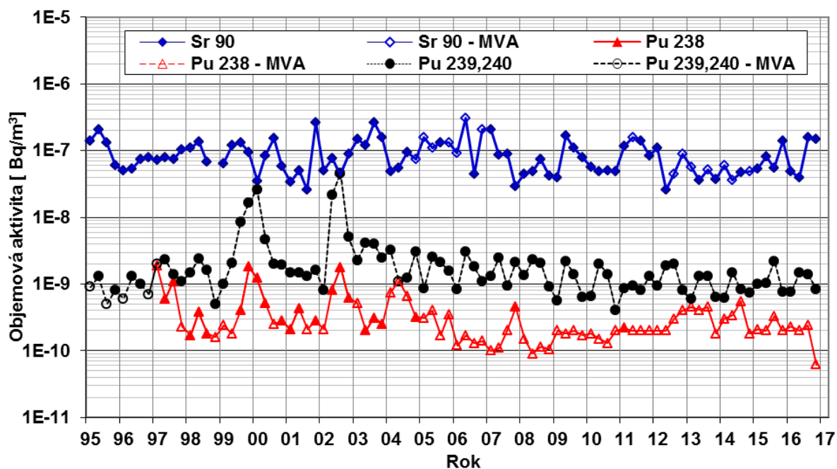
Obr. 8b Objemová aktivita ^{90}\text{Sr} , ^{238}\text{Pu} , ^{239,240}\text{Pu} v aerosolu v ovzduší od roku 1995 – MMKO Praha (vzorkování a měření SÚRO Praha)
