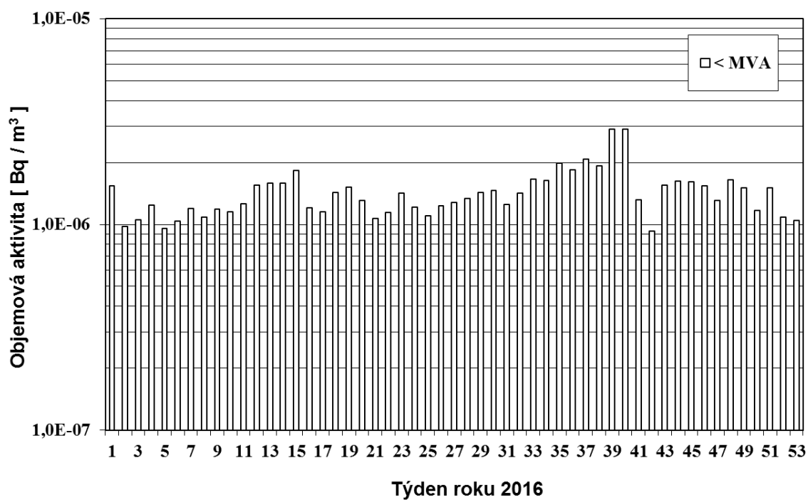
Obr. 17b Objemová aktivita 137 Cs ve vzdušném aerosolu v roce 2016 ve vzorcích odebraných na stanicích v okolí a v areálu JE Temelín (odběr a měření LRKO JE Temelín)
