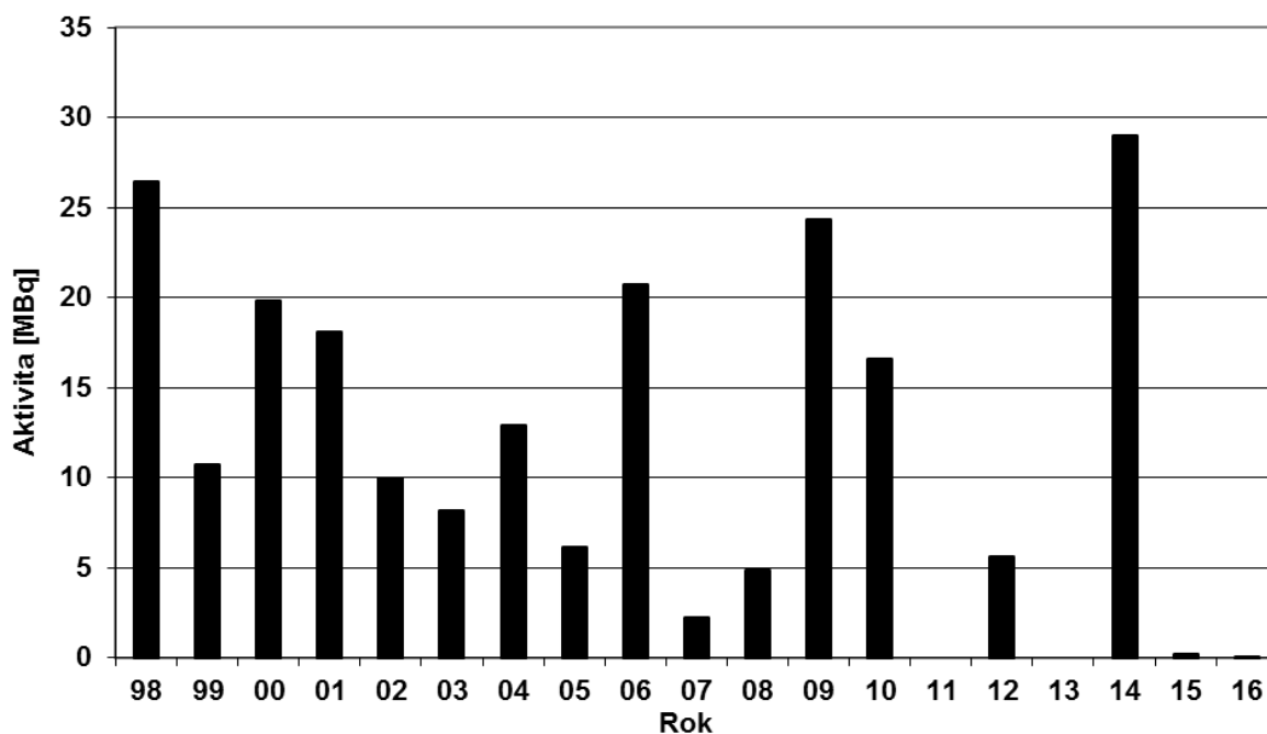
Obr. 15b Bilance plyných výpustí - ^{131}\text{I} z odběrů ve ventilačním komínu ÚJV Řež v období 1998 – 2016 (celkový roční limit aktivity je 20 000 [MBq]), (vzorkování a měření ÚJV Řež)
