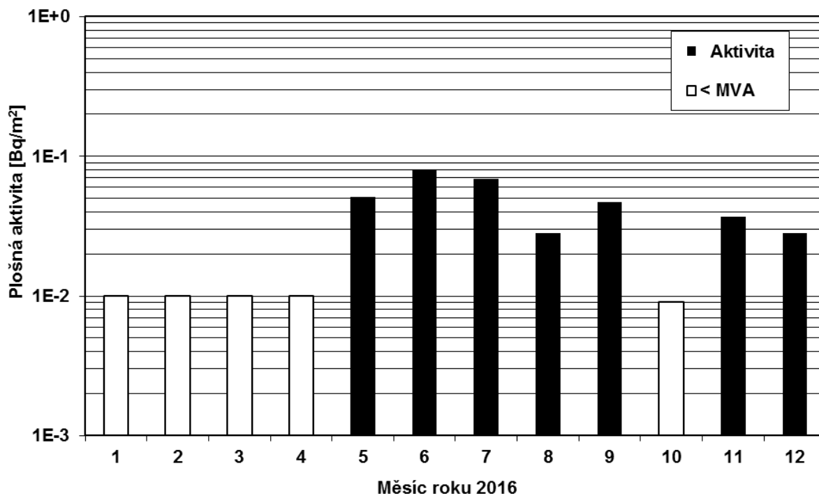
Obr. 10a Plošná aktivita ^{137}\text{Cs} ve spadech v roce 2016, měsíční hodnoty – MMKO Ostrava (vzorkování a měření SÚRO Ostrava)
