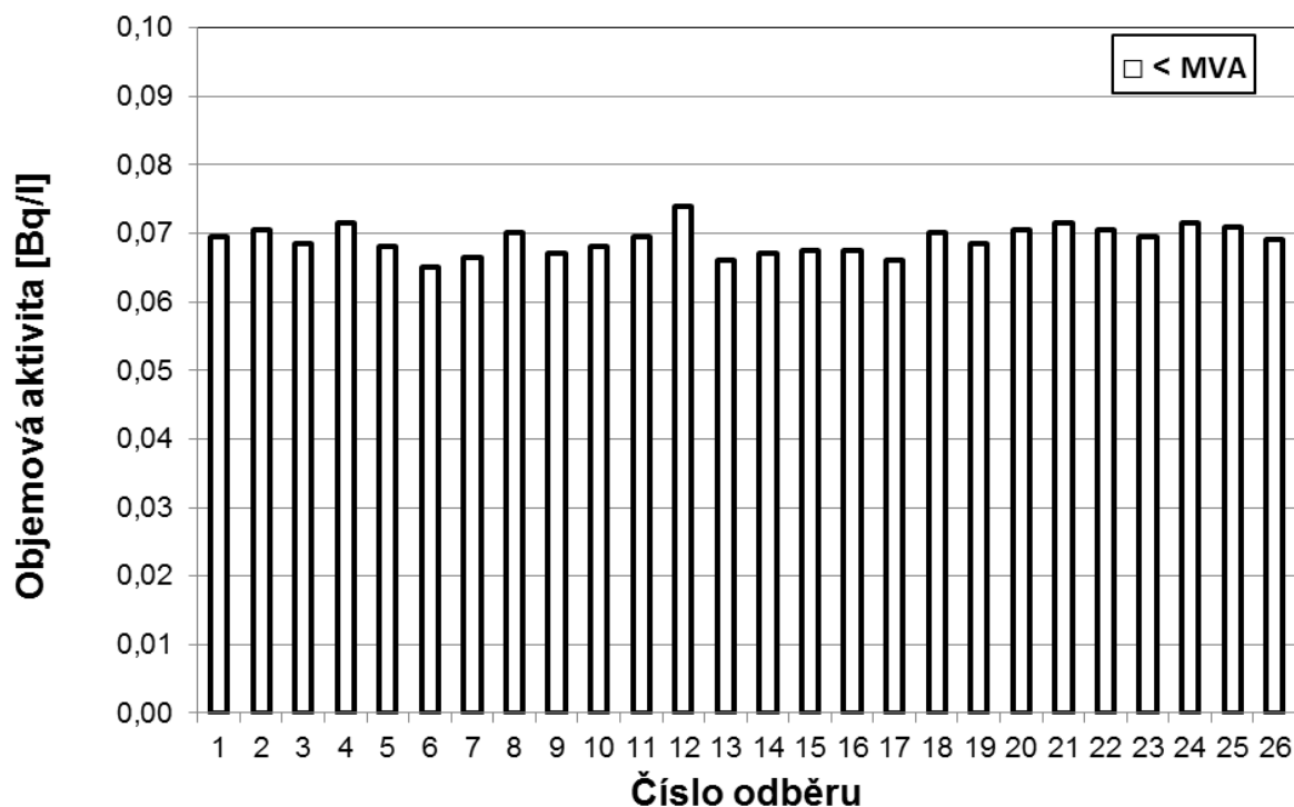
Obr. 18b Objemová aktivita ^{137}\text{Cs} v mléce v roce 2016 ve vzorcích odebraných v kravínech v ZHP JE Temelín (odebírání se jednou za 14 dní; odběr a měření LRKO JE Temelín)
