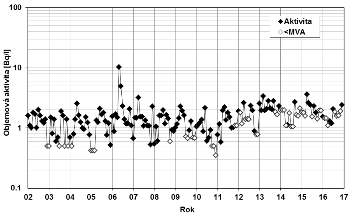
Obr. 11b Objemová aktivita ^3\text{H} ve srážkách od roku 2002, měsíční odběry – MMKO Praha (vzorkování a měření SÚRO Praha)
