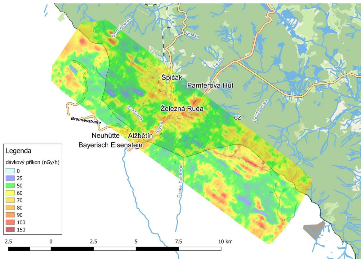
Obr. 5 Výsledky leteckého přeshraničního (CZ-DE) monitorování v okolí Železné Rudy.
