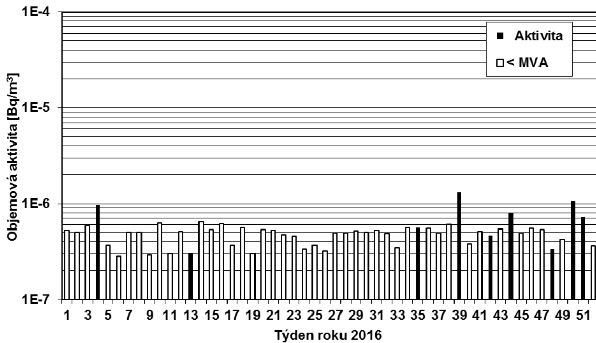
Obr. 7a Objemová aktivita ^{137}\text{Cs} v aerosolu v ovzduší v roce 2016 – MMKO Kamenná (vzorkování MMKO Kamenná, měření SÚRO Ostrava)
