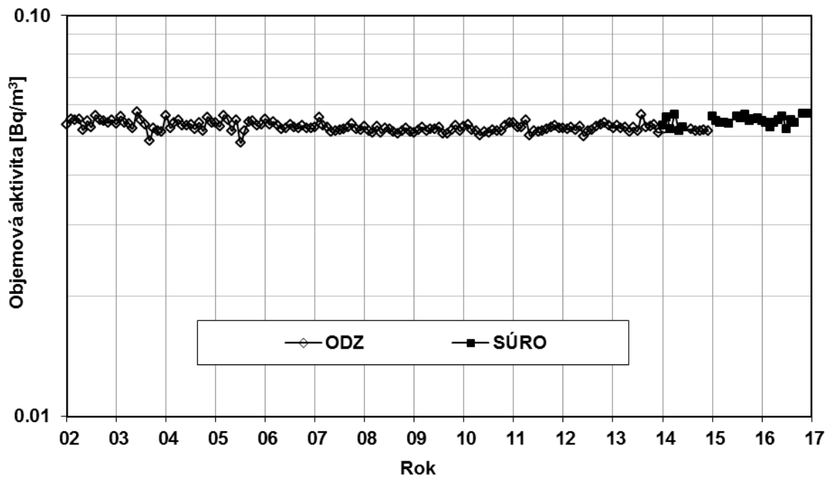
Obr. 9b Objemová aktivita ^{14}\text{C} v ovzduší ve formě \text{CO}_2 , měsíční průměry – MMKO Praha – (do 2013 vzorkování a měření ODZ ÚJF AV, od 2014 vzorkování a měření i SÚRO Praha)
