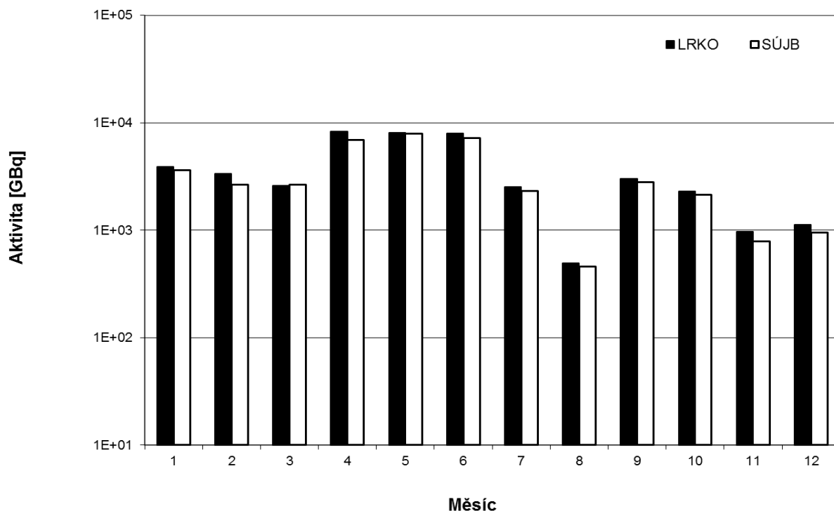
Obr. 20a Celková aktivita ^3\text{H} vypouštěná do vodoteče z JE Temelín v roce 2016 (porovnání hodnot naměřených SÚJB a LRKO provozovatele, odběr JE Temelín, měření RC SÚJB Brno a LRKO JE Temelín)
