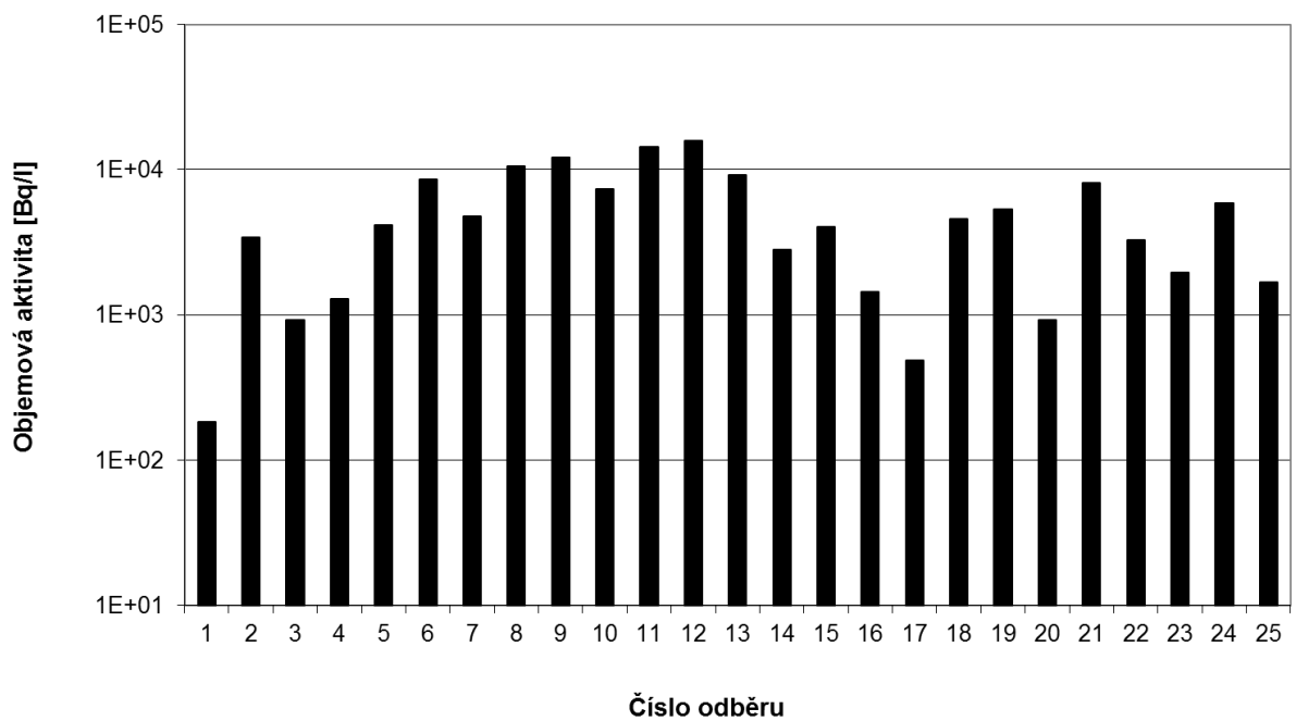
Obr. 20b Objemová aktivita ^3\text{H} v odpadním kanále JE Temelín v roce 2016 (čtrnáctidenní slévané vzorky, odběr ETE, měření RC SÚJB Brno)
