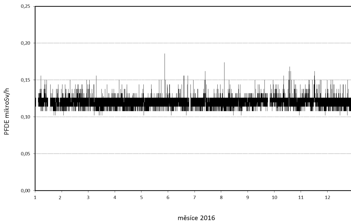
Obr. 2e Příkon fotonového dávkového ekvivalentu (PFDE) - SVZ Hradec Králové (měřicí místo RC SÚJB)
