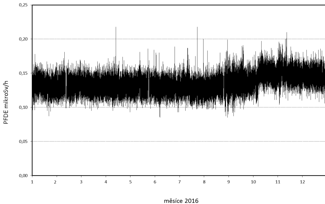
Obr. 16c Příkon fotonového dávkového ekvivalentu (PFDE) - SVZ TDS2 Kordula (měřicí místo JE Dukovany)
