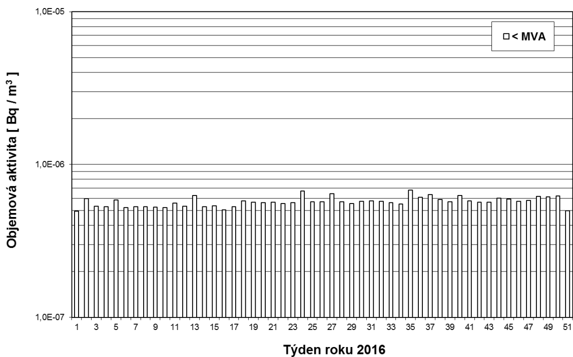
Obr. 17a Objemová aktivita 137 Cs ve vzdušném aerosolu v roce 2016 ve vzorcích odebraných na stanicích v okolí a v areálu JE Dukovany (odběr a měření LRKO JE Dukovany)
