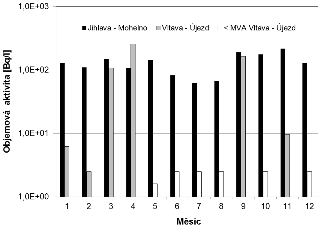
Obr. 21 Objemová aktivita 3 H v řece Jihlavě (profil Mohelno) a v řece Vltavě (profil Újezd) v roce 2016 (odběr RC SÚJB Brno a RC SÚJB Č. Budějovice, měření RC SÚJB Brno)
