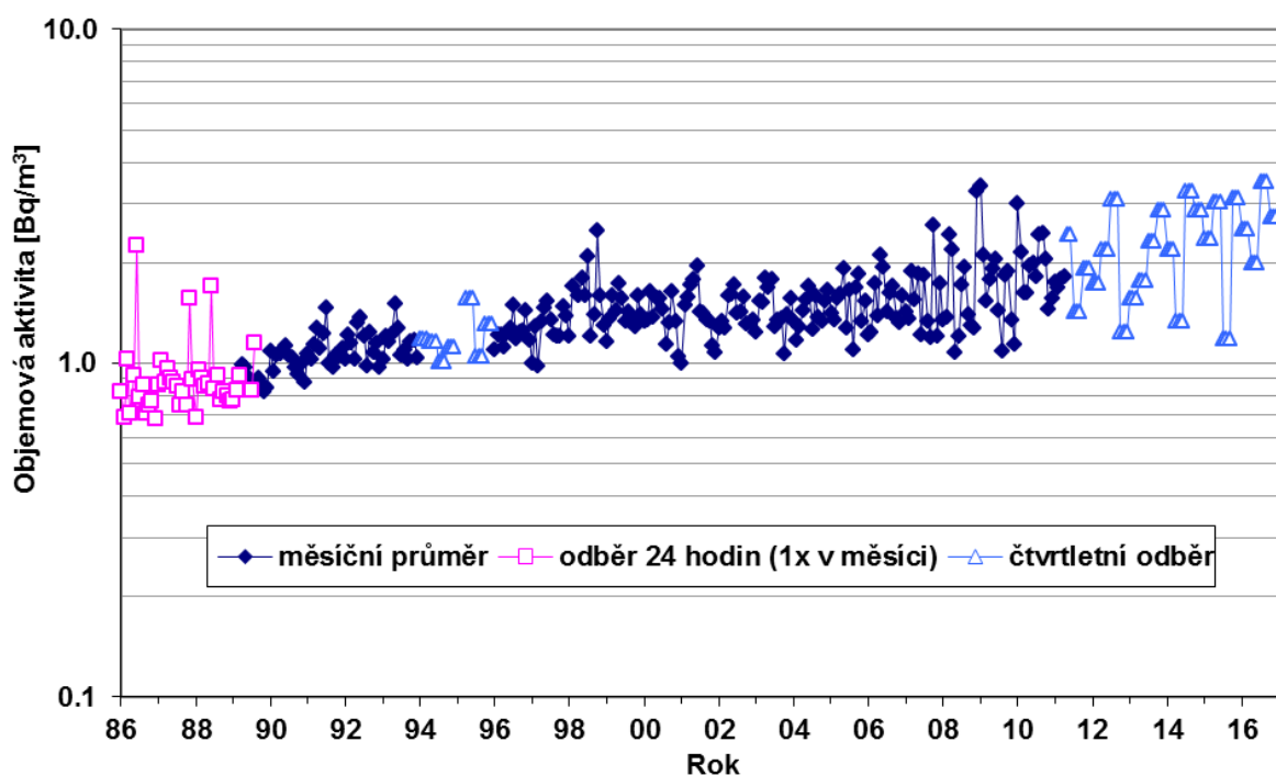
Obr. 9a Objemová aktivita ^{85}\text{Kr} v ovzduší – MMKO Praha (vzorkování a měření ODZ ÚJF AV ČR)
