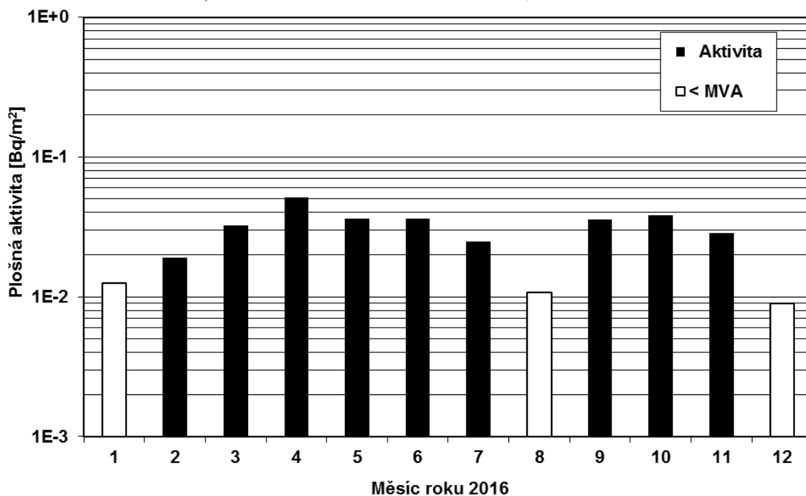
Obr. 10b Plošná aktivita ^{137}\text{Cs} ve spadech v roce 2016, měsíční hodnoty – MMKO Hradec Králové (vzorkování a měření SÚRO Hradec Králové)
